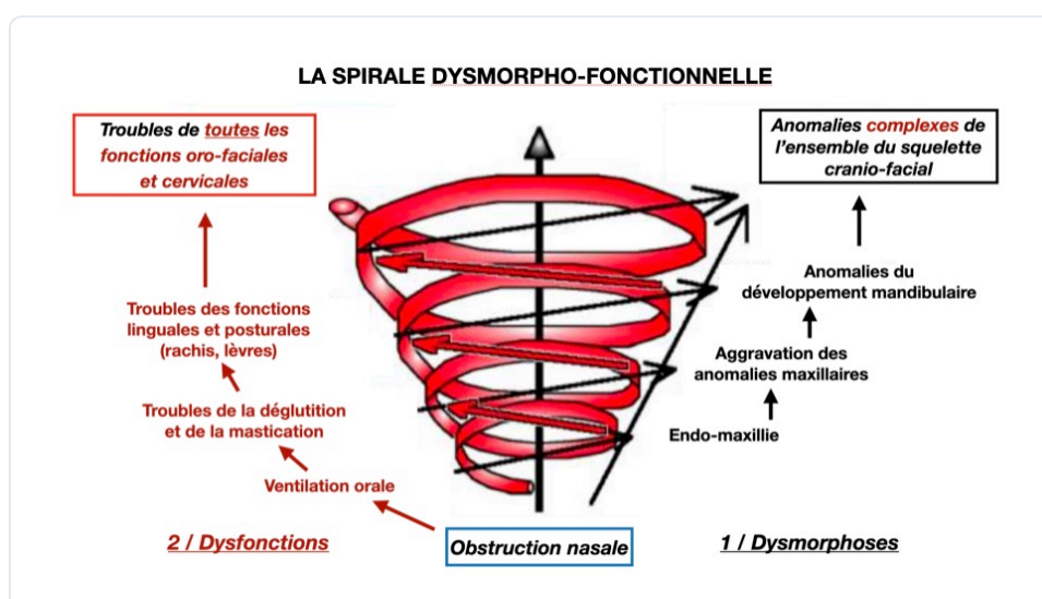
Figure 7. Cascade dysmorpho-fonctionnelle.
